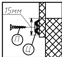
Крепление задней стенки к детали №109 (комплект №10)
