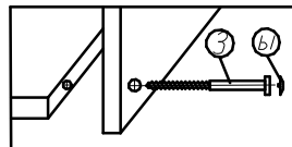
Крепление винта саморезного (комплект №19)
