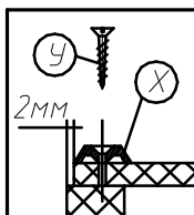
Крепление штанги (комплект №6)
