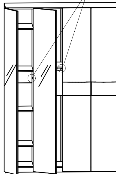
K-Push крепление к деталям №105, №99
